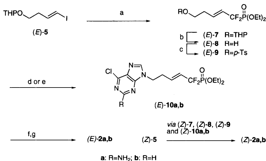
Scheme 1. Reagents: (a) BrZnCF 2 P(O)(OEt) 2 ( 6 ), CuBr, DMF, 25 °C; (b) p -TsOH, MeOH; (c) p -TsCl, Et 3 N, CH 2 Cl 2 ; (d) 2-amino-6-chloropurine, K 2 CO 3 , DMF; (e) 6-chloropurine, K 2 CO 3 , DMF; (f) TMSBr, CH 2 Cl 2 ; (g) H 2 O.
