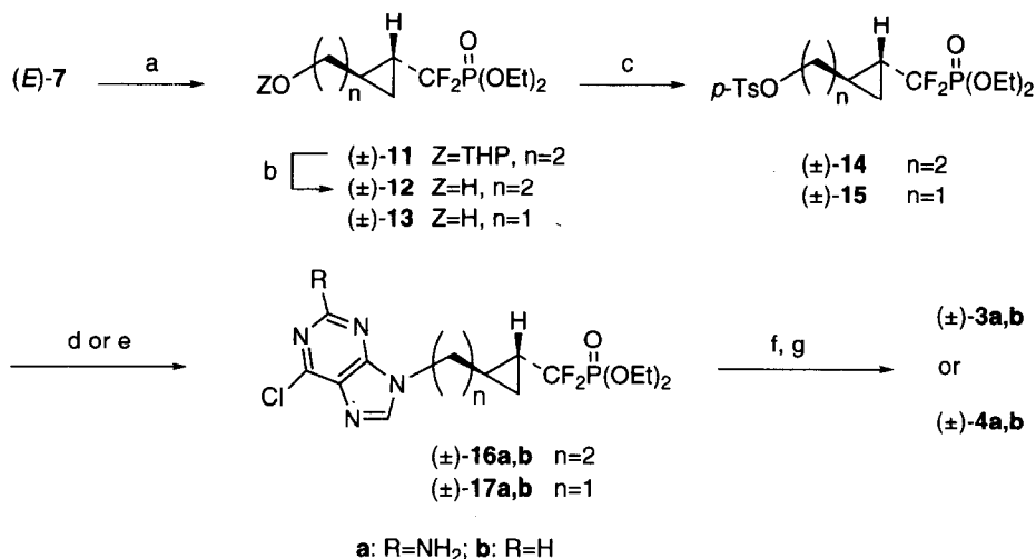
Scheme 2. Reagents: (a) CH 2 N 2 , Pd(OAc) 2 , ether; (b) p -TsOH, MeOH; (c) p -TsCl, Et 3 N, CH 2 Cl 2 ; (d) 2-amino-6-chloropurine, K 2 CO 3 , DMF; (e) 6-chloropurine, K 2 CO 3 , DMF; (f) TMSBr, CH 2 Cl 2 ; (g) H 2 O.
